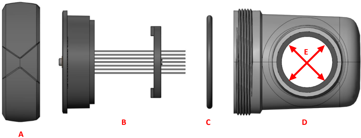
Vista despiezada del montaie:
