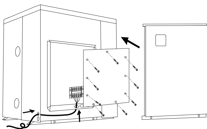
(4) Installer le couvercle du boîtier électrique
