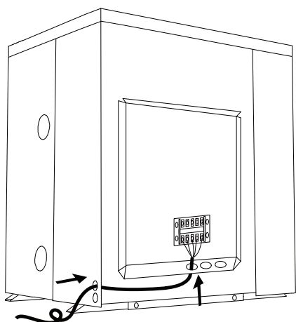
(5) Installer le panneau avant
