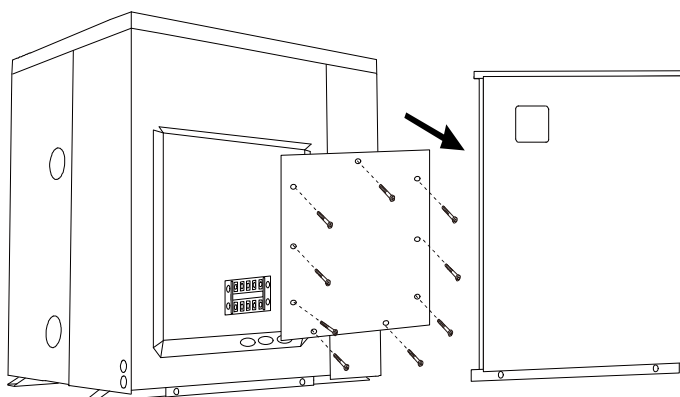
(2) Retirer le couvercle du boîtier électrique
